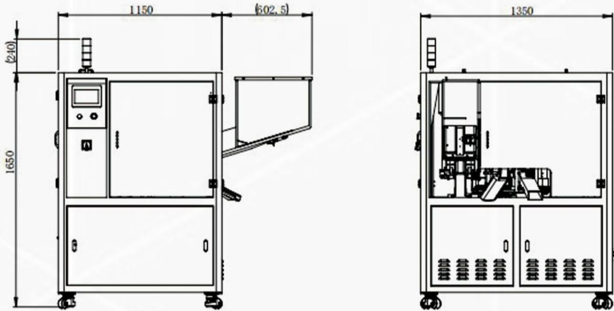
平面图/Plan view
